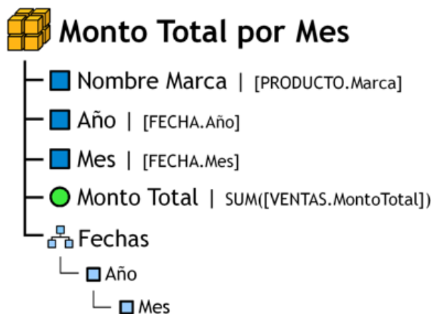
Figura 5.37: Cubo 2, ejemplo.
