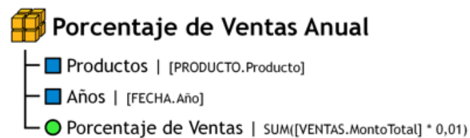
Figura 5.38: Cubo 3, ejemplo.
