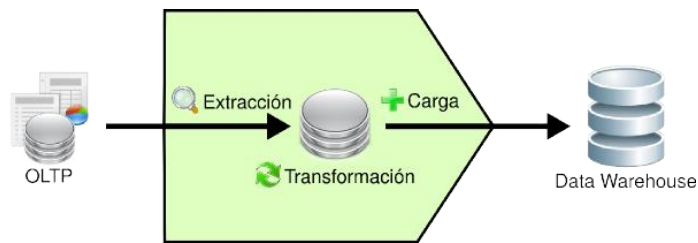
Figura 3.8: Proceso ETL.
