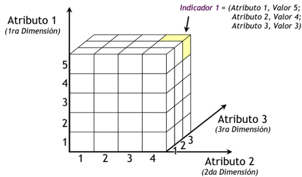
Figura 3.13: Cubo multidimensional.
