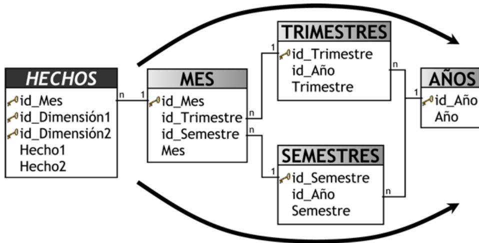
Figura 6.2: Trayectoria cíclica.
