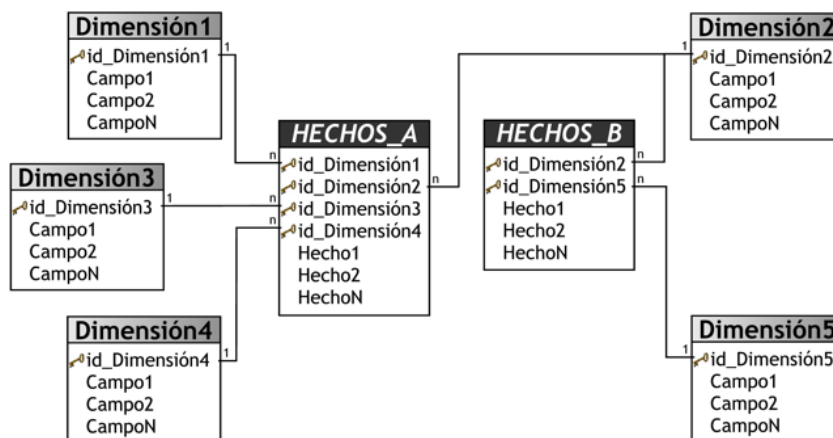
Figura 3.19: Esquema Constelación.
