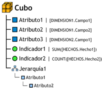
Figura 3.22: Cubo estándar.
