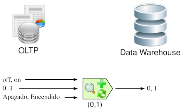
Figura 3.4: Transformación: codificación.
