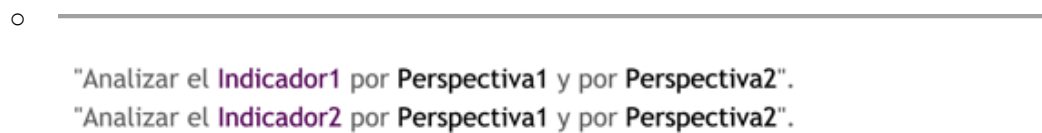
Figura 5.21: Caso 3, preguntas.
