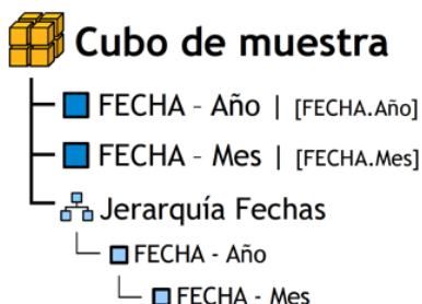
Figura 3.14: Jerarquía Fechas.
