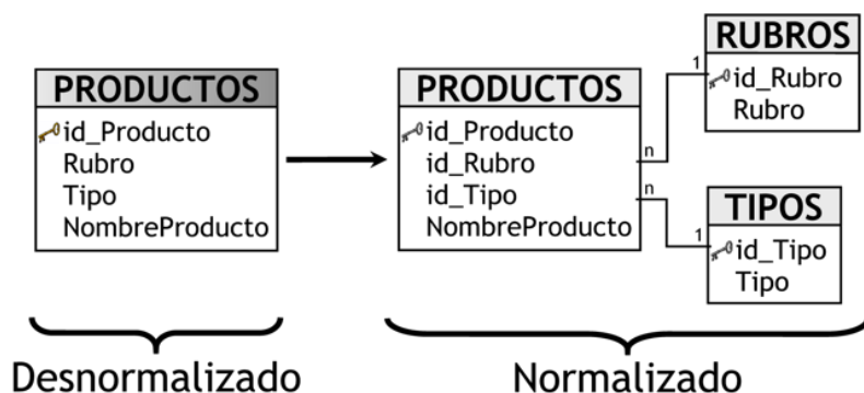
Figura 3.17: Desnormalización.
