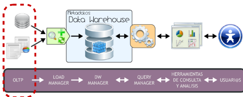
Figura 3.2: OLTP
