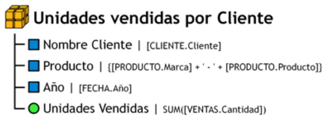
Figura 5.36: Cubo 1, ejemplo
