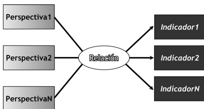
Figura 5.4: Modelo Conceptual.
