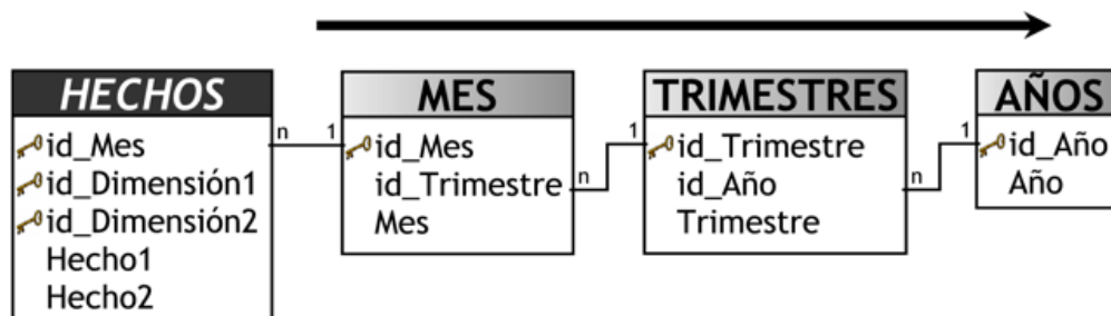
Figura 6.1: Trayectoria acíclica.
